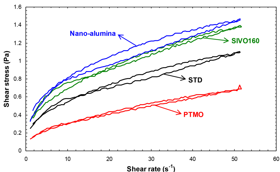
Figura 9. Curvas de flujo de la suspensión de esmalte para vajilla incorporando el tratamiento del cuarzo con diferentes aditivos.
