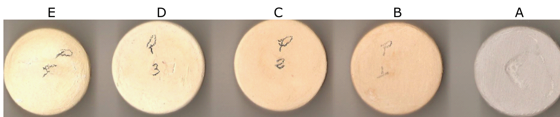
A – Muestra antes de la sinterización; B – muestra sinterizada a 850°C; C – Muestra sinterizada a 900°C; D – muestra sinterizada a 1000°C; E – Muestra sinterizada a 1100°C.
