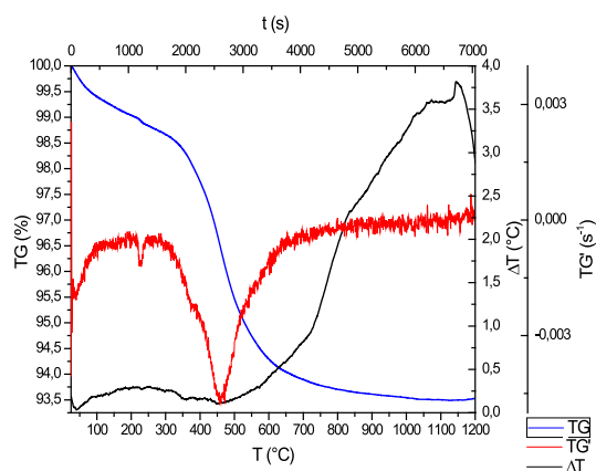
Figura 11. Curvas de ATD – TG – DTG Cumbre-Santander
