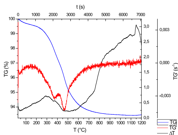
Figura 14. Curvas de ATD – TG – DTG material Los Pozos Arcabuco
