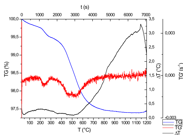
Figura 8. Curvas de ATD - TG - DTG Abejorral - Caldas
