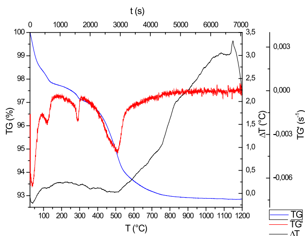
Figura 2. Curvas de ATD – TG – DTG formación Amagá
