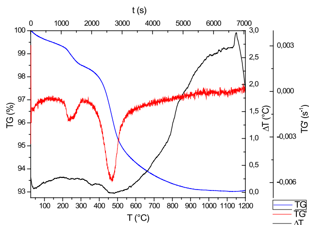
Figura 5. Curvas de ATD – TG – DTG La Soledad-Amalfi
