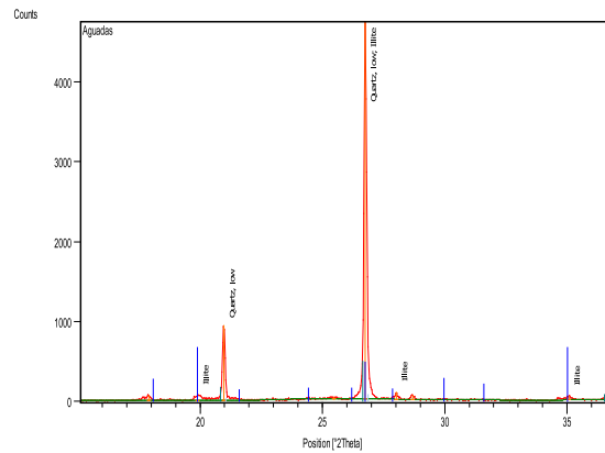
Figura 7. Difractograma Abejorral - Caldas
