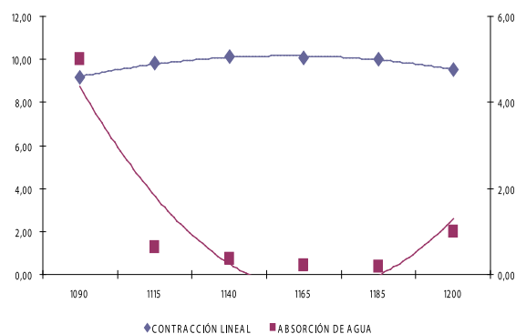
Figura 12. Curva de gresificación Cumbre-Santander
