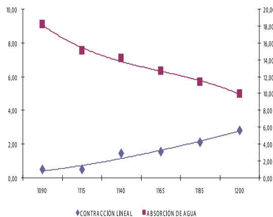
Figura 9. Curva de gresificación Abejorral - Caldas
