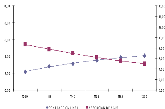
Figura 15. Curva de gresificación material Arcabuco
