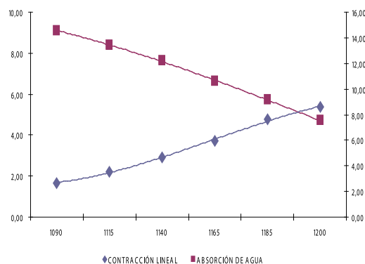
Figura 6. Curva de gresificación La Soledad-Amalfi
