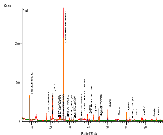
Figura 4. Difractograma La Soledad-Amalfi
