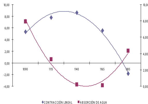
Figura 3. Curva de gresificación formación Amagá
