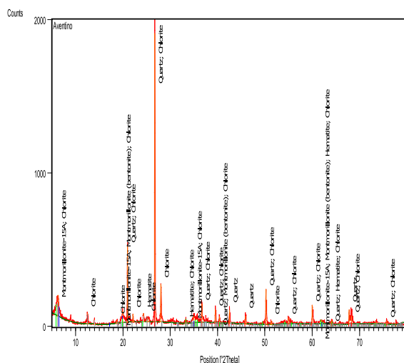
Figura 1. Difractograma formación Amaqá
