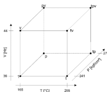
Figura 5. Diseño Experimental 2 3 . Vista geométrica.
