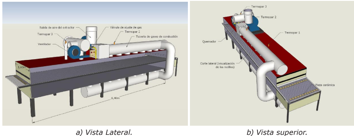
Figura 3. Esquema del secadero utilizado.
