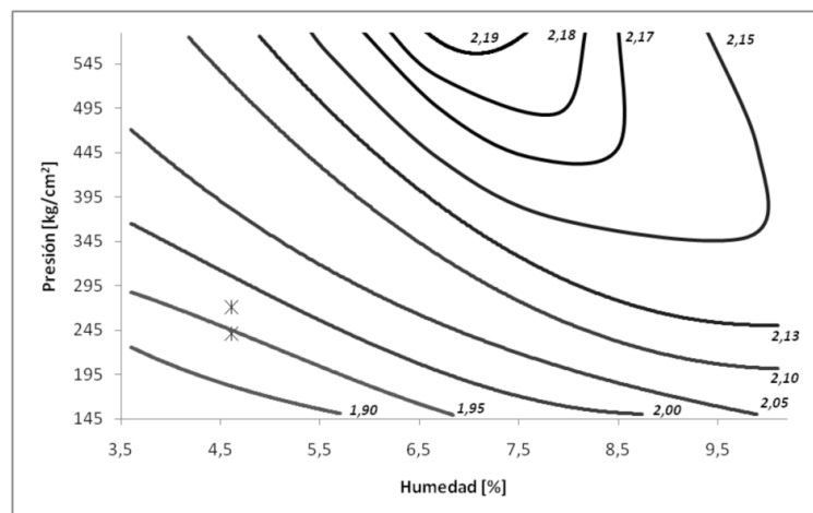
Figura 4. Diagrama de isocompactación 2 con condiciones de operación.
