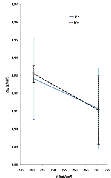
Figura 8. Gráfico de Interacción V*P .
