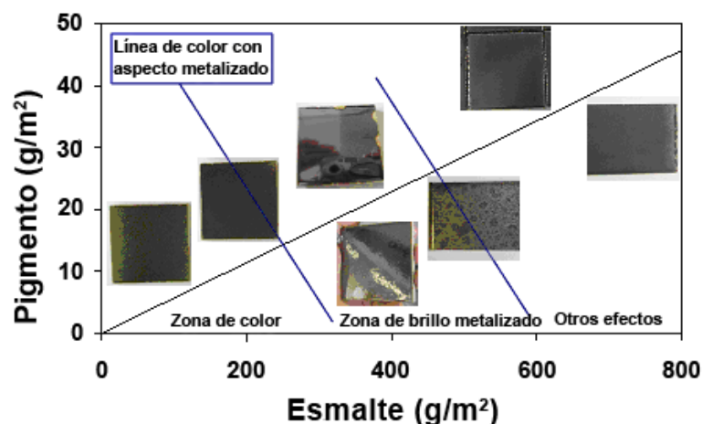
Figura 3. Diferentes efectos conseguidos con la incorporación de nanopartículas de cobre al esmalte a través de sepiolita.
