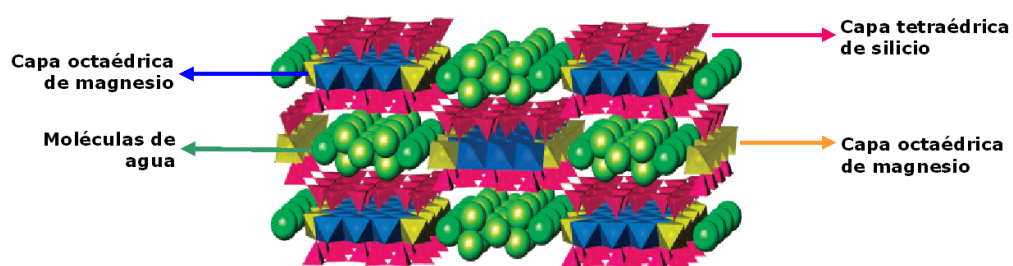
Figura 1. Estructura de la arcilla sepiolita: Tetraedros de sílice, octaedros de magnesio y agua zeolítica.
