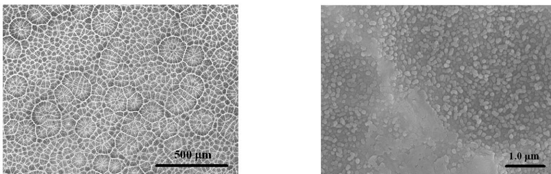
Figura 5. a) Imagen MOLP de la microestructura de aspecto celular presente en esmalte con aspecto metalizado. b) Imagen MEB de la nanoestructura generada mediante descomposición espinodal en la superficie de la microestructura de aspecto celular.
