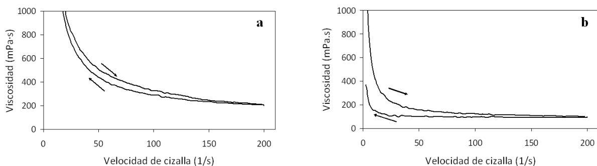
Figura 2. Curvas reológicas de a) esmalte cristalino habitual b) esmalte con sepiolita con nanopartículas metálicas.
