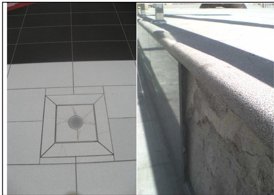
Figura 1. Ejemplos de patologías de integración de plaquetas porcelánicas con materiales cementantes: a) Arqueta en pavimento del aeropuerto de Dreden, Alemania y b) no-relación o ausencia de integración con material cementicio en paseo peatonal de una playa de la costa mediterránea (fotos originales de J. Ma. Rincón, 2009).
