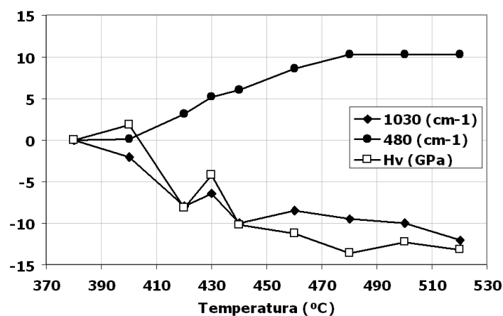
Figura 2. Variación de las posiciones Raman y de la microdureza de fritas con T_r .
