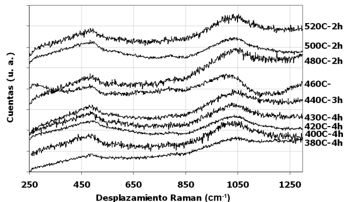
Figura 1. Espectros Raman de Fritas tratadas.
