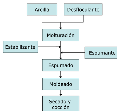
Figura 1. Esquema de la preparación de las espumas cerámicas por incorporación de fase gaseosa por agitación enérgica.
