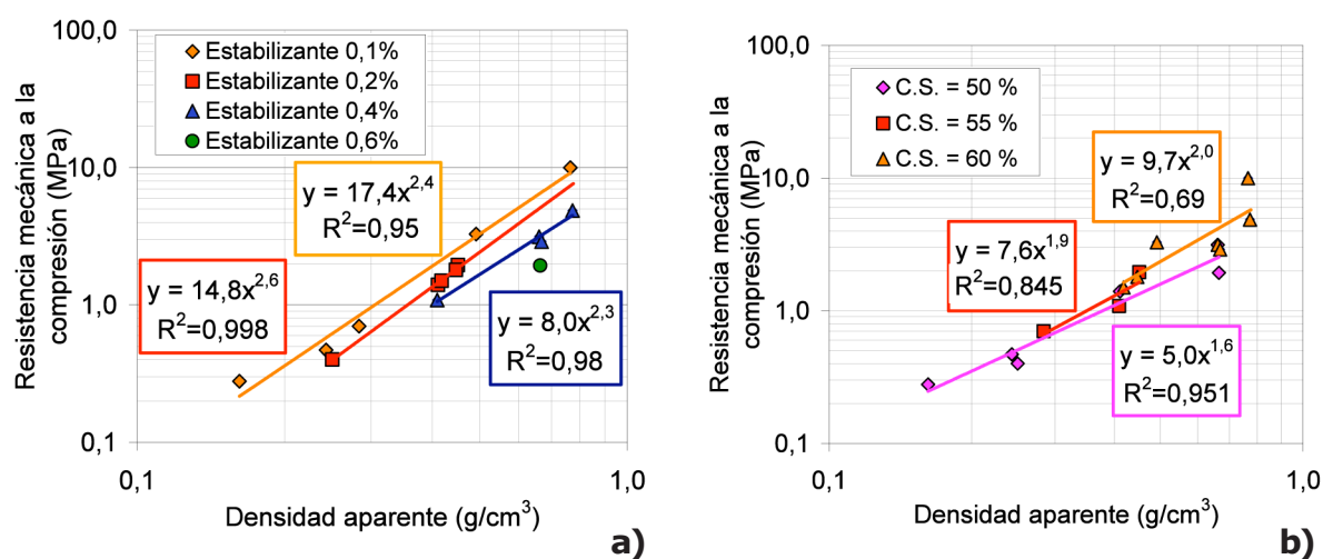
Figura 3, 3a y 3b. Relación entre la resistencia a la compresión y la densidad aparente de las espumas cocidas para diferentes contenidos de estabilizante y de sólidos.
